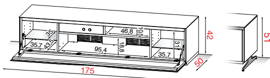
Avec pieds H. 51 (Option page 72)
