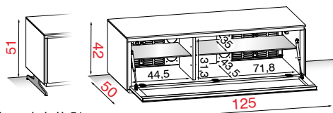
Avec pieds H. 51 (Option page 20)
