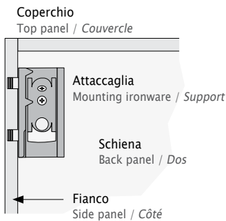
VISTA POSTERIORE REAR VIEW / VUE ARRIÈRE
