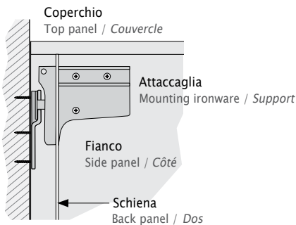
VISTA LATERALE SIDE VIEW / VUE LATÉRALE
