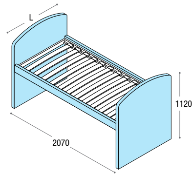
Letto fisso TRIS Bed fixed / Lit fixe
