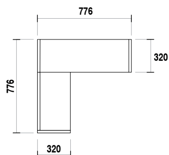
Ingombro angoli a giorno Dimensions open corner module Encombrement des éléments angles ouverts
