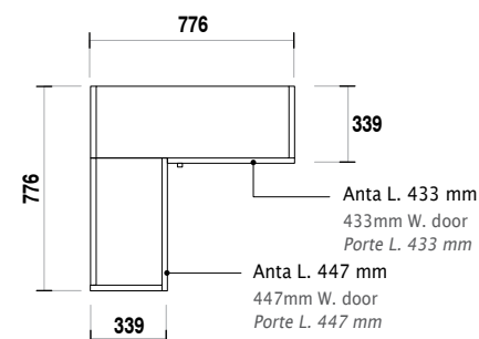
Ingombro angoli con ante Dimensions corner module with doors Encombrement des éléments angles avec portes
