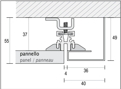
Cremagliera finale Final slotted rail / Crémaillère finale
